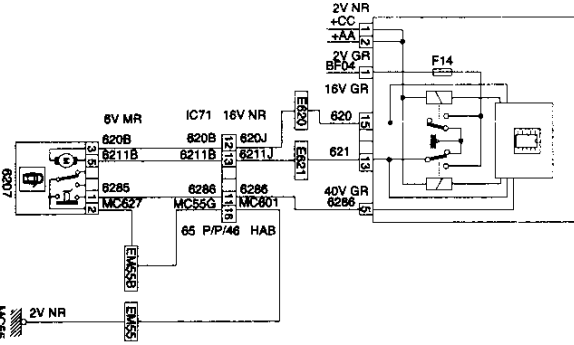
6207 CONJUNTO CERRADURA PUERTA DELANTERA DERECHA (PACK 1)
