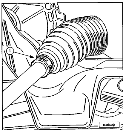
Quitar la abrazadera (1).
