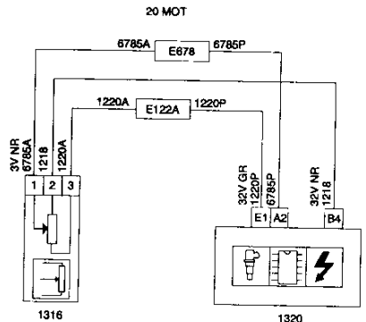
1316 CAPTADOR DE POSICIÓN MARIPOSA (MOTOR EW10J4 - ANTICONTAMINACIÓN L4)
