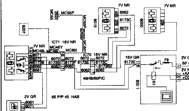
6005 CONTACTOR ELEVALUNAS ACOMPAÑANTE PUERTA ACOMPAÑANTE
