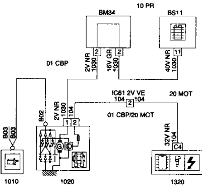
1020 ALTERNADOR (MOTOR EW10J4 - ANTICONTAMINACIÓN L4)
