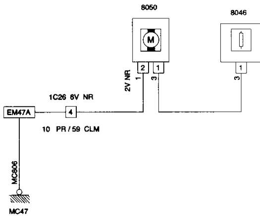
8050 MOTOR VENTILADOR (SI SEPARADO)
