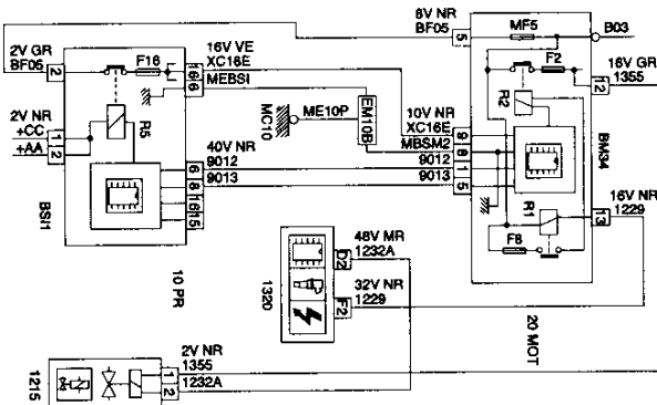
1215 ELECTROVÁLVULA DE PURGA CÁNISTER
