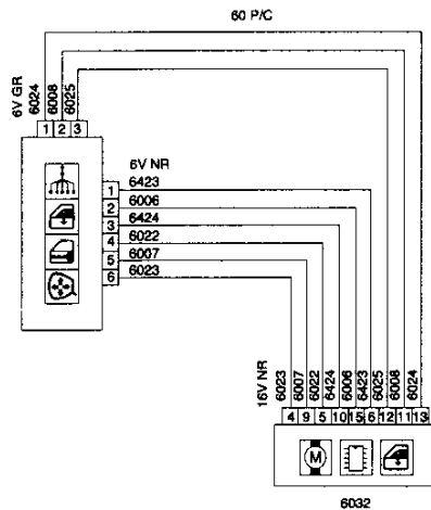
6036 PLATINA DE MANDO ELEVAVINAS/RETRO PUERTA CONDUCTOR
