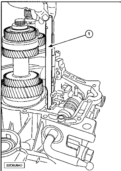
Montar el eje de horquilla de 5ª (1).
