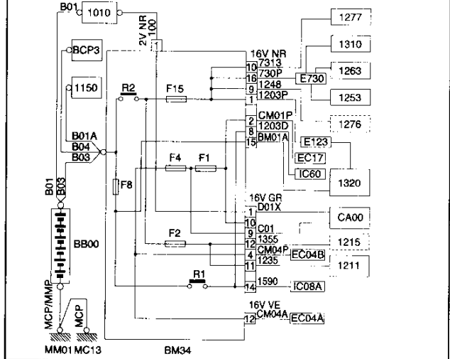
BM34 CAJETÍN DE SERVICIO MOTOR 34 FUSIBLES (MOTOR DW10TD CALCULADOR SIEMENS PARA DW10)
