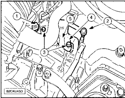
Quitar el captador régimen motor (1).
