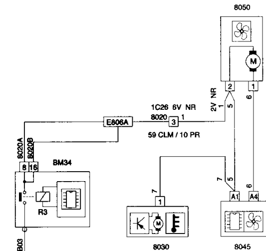
8050 MOTOR VENTILADOR (SI SEPARADO) (AIRE ACONDICIONADO REGULADO)
