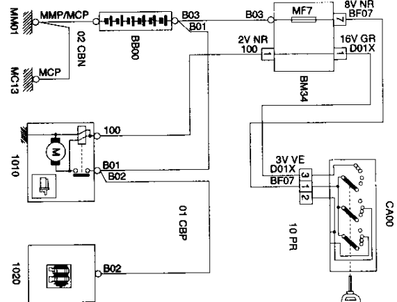
BB00 BATERÍA
