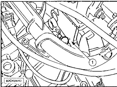
Quitar el captador régimen motor (1).
