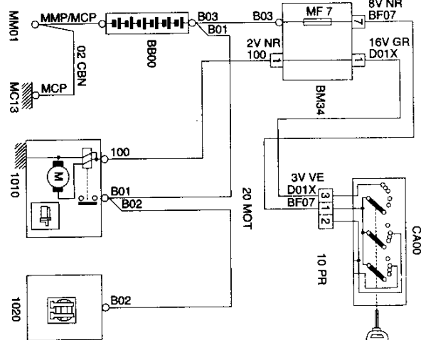
BB00 BATERÍA (MOTOR TU3JP)
