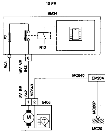
5405 BOMBA LAVAFAROS
