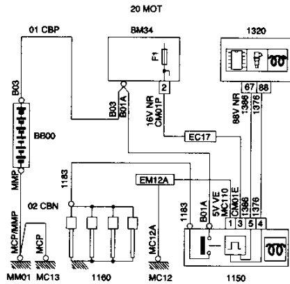
1150 CAJETÍN DE PRECALENTAMIENTO (MOTOR DW10TD CALCULADOR BOSCH PARA DW10/DW12)
