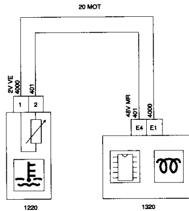
1220 CAPTADOR TEMPERATURA AGUA MOTOR (MOTOR DW10TD CALCULADOR SIEMENS PARA DW10)
