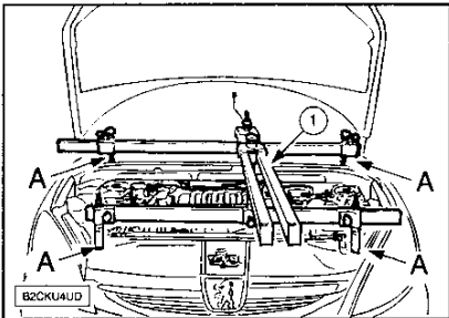
Montar la travesía de sujeción GMP (1).
