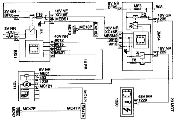
1211 AFORADOR DE CARBURANTE (MOTOR DW10TD SIEMENS PARA DW10)
