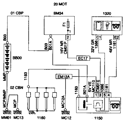
1150 CAJETÍN DE PRECALENTAMIENTO (MOTOR DW10TD CALCULADOR SIEMENS PARA DW10)
