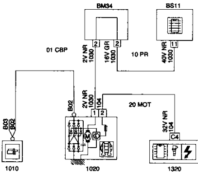
1020 ALTERNADOR (MOTOR TU5JP VERSIÓN EUROPA)
