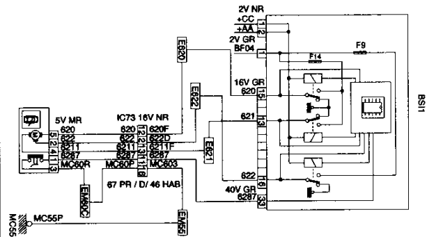
6217 CONJUNTO CERRADURA PUERTA TRASERA DERECHA (SUPERCONDENACIÓN - PACK 3)
