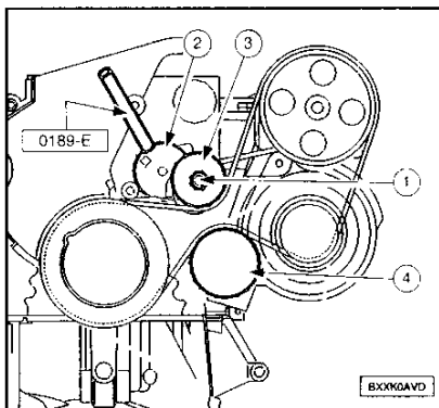
Motor EW10J4.
