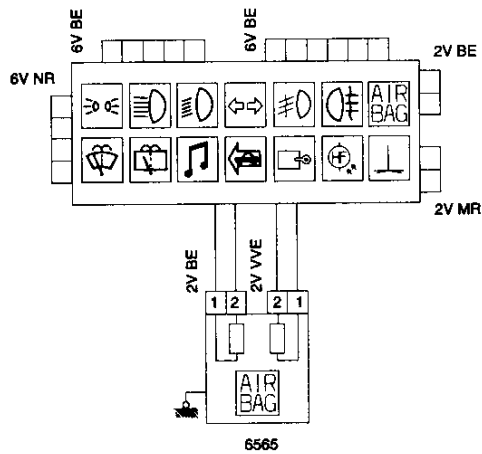
6565 MÓDULO COJÍN INFLABLE CONDUCTOR
