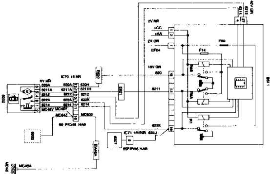
6202 CONJUNTO CERRADURA PUERTA DELANTERA IZQUIERDA (SUPERCONDENACIÓN 3 PUERTAS)
