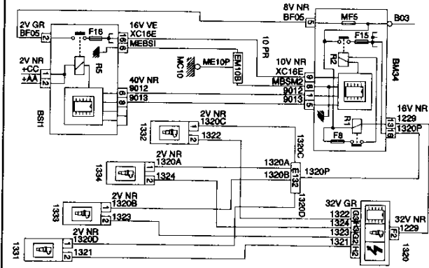
1334 INYECTOR CILINDRO N° 4 (MOTOR EW10J4 - ANTICONTAMINACIÓN L4)
