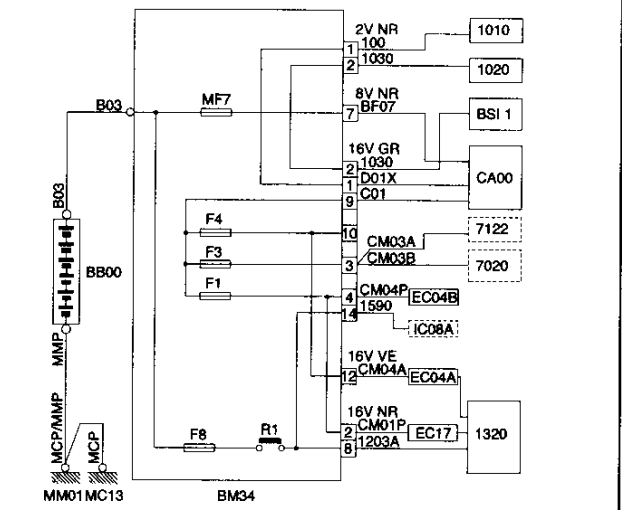
BM34 CAJETÍN DE SERVICIO MOTOR 34 FUSIBLES
