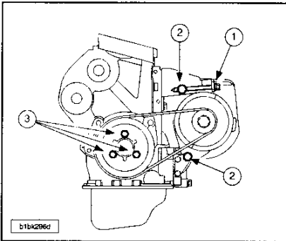
Motores TU3JP y TU5JP4.
