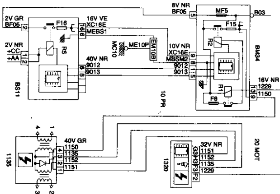
1135 BOBINA DE ENCENDIDO (MOTOR TU3JP)
