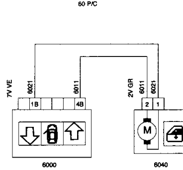
6040 MOTOR ELEVAVINAS DELANTERO (LADO IZQUIERDO)
