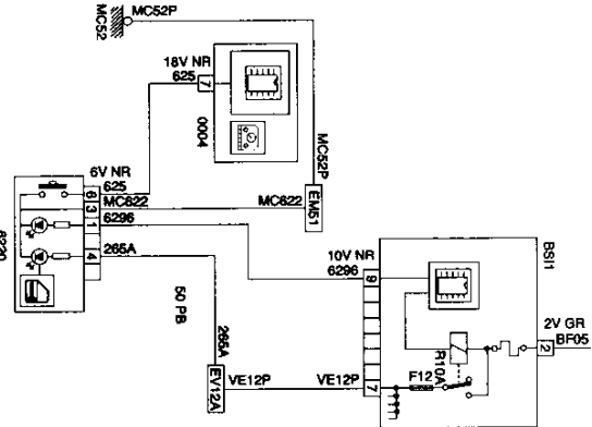
6220 CONTACTOR DE CONDENACIÓN PUERTAS
