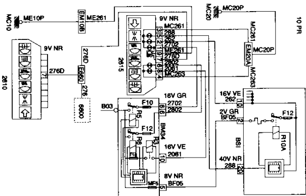
2615 FARO DERECHO
