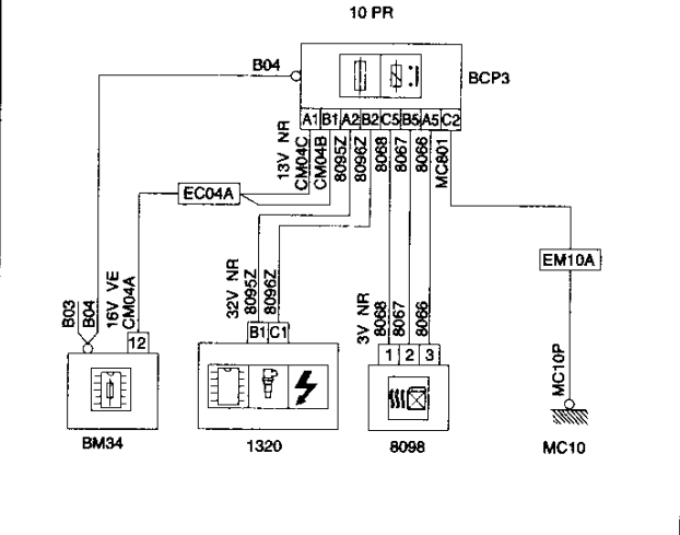
BM34 CAJETÍN DE SERVICIO MOTOR 34 FUSIBLES
