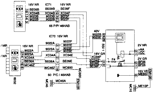
6032 MOTOR + CAJETÍN ELEVAVINAS DELANTERO SECUENCIAL CONDUCTOR
