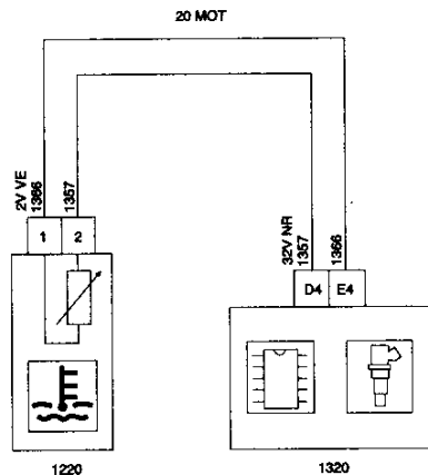
1220 CAPTADOR TEMPERATURA AGUA MOTOR (MOTOR EW10J4 - ANTICONTAMINACIÓN L4)
