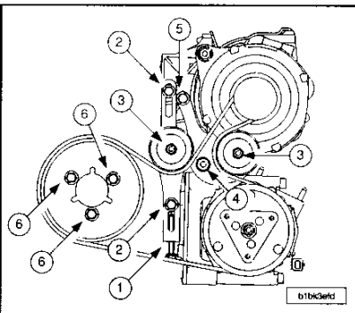
Aire acondicionado, motor TU3JP.
