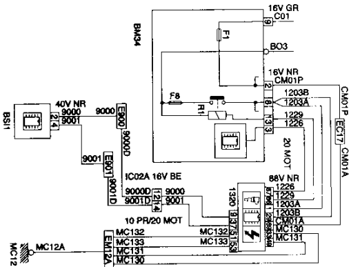
1320 CALCULADOR MOTOR (MOTOR DW10TD CALCULADOR BOSCH PARA DW10/DW12)
