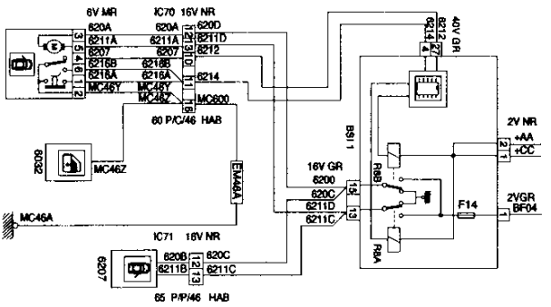
6202 CONJUNTO CERRADURA PUERTA DELANTERA IZQUIERDA (CALCULADOR PLATINA DE PUERTA CONDUCTOR - 3 PUERTAS)
