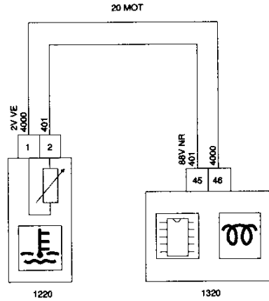
1220 CAPTADOR TEMPERATURA AGUA MOTOR (MOTOR DW10TD CALCULADOR BOSCH PARA DW10/DW12)
