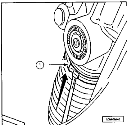
Quitar la abrazadera (1).
