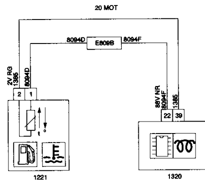
1221 TERMISTENCIA GASOIL (MOTOR DW10TD CALCULADOR BOSCH PARA DW10/DW12)
