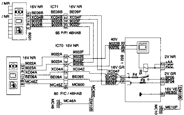
6031 MOTOR + CAJETÍN ELEVAVINAS DELANTERO SECUENCIAL ACOMPAÑANTE
