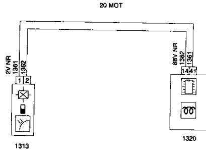
1313 CAPTADOR RÉGIMEN MOTOR (MOTOR DW10TD CALCULADOR SIEMENS PARA DW10)
