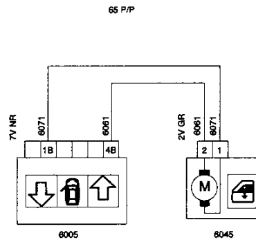
6045 MOTOR ELEVAVINAS DELANTERO (LADO DERECHO)
