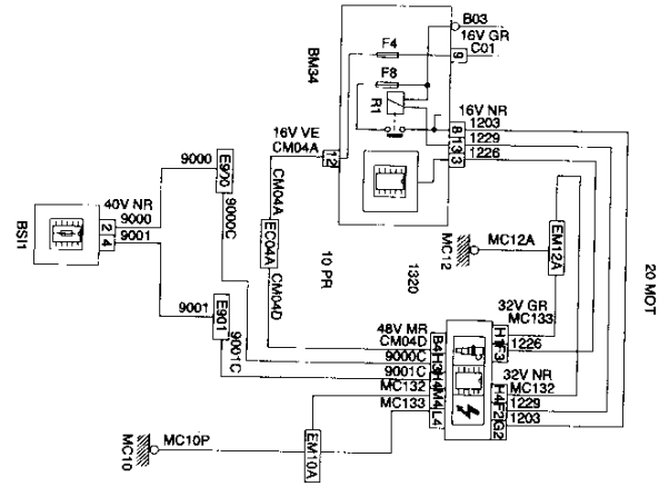
1320 CALCULADOR MOTOR (MOTOR TU5JP4 VERSIÓN EUROPA)
