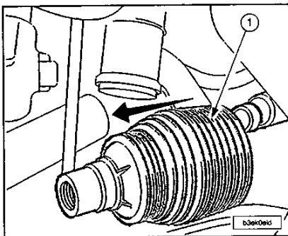
Sacar el guardapolvos de estanqueidad (1).
