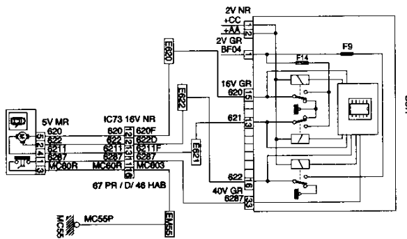
6217 CONJUNTO CERRADURA PUERTA TRASERA DERECHA (SUPERCONDENACIÓN)
