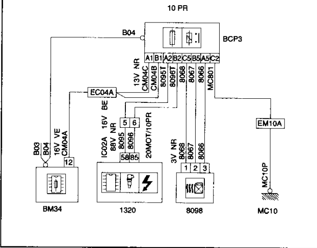
BCP3 CAJETÍN CONMUTACIÓN PROTECCIÓN 3º RELÉ (MOTOR DW10TD CALCULADOR SIEMENS PARA DW10)
