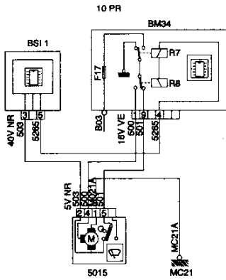
5015 MOTOR LIMPIAPARABRISAS
